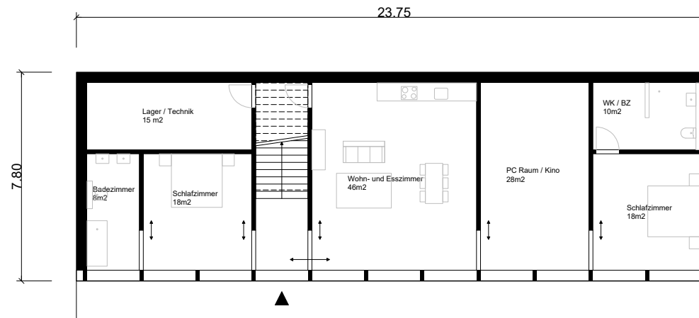
1. Untergeschoss
