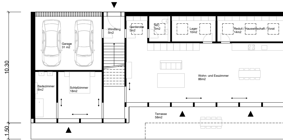
Erdgeschoss
