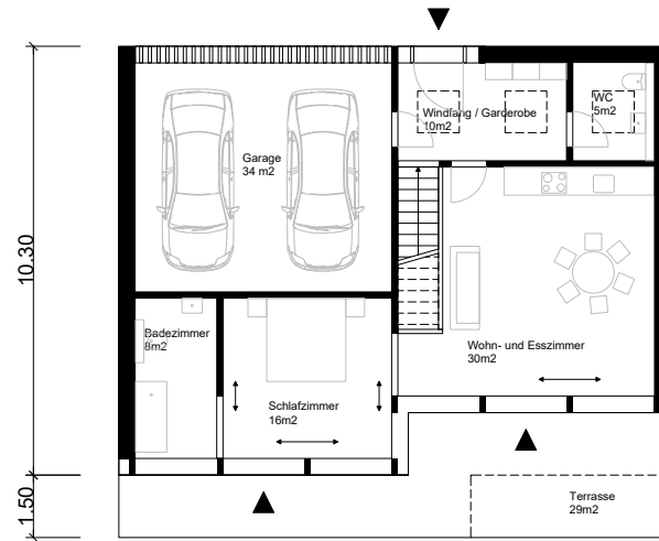
Erdgeschoss
