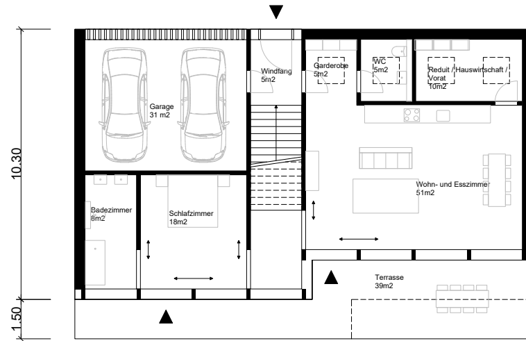
Erdgeschoss
