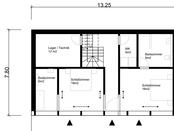
1. Untergeschoss
